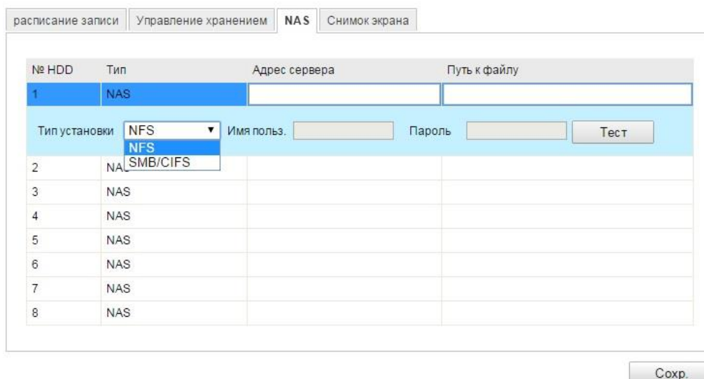
Рисунок 7-1 Добавление сетевого диска
